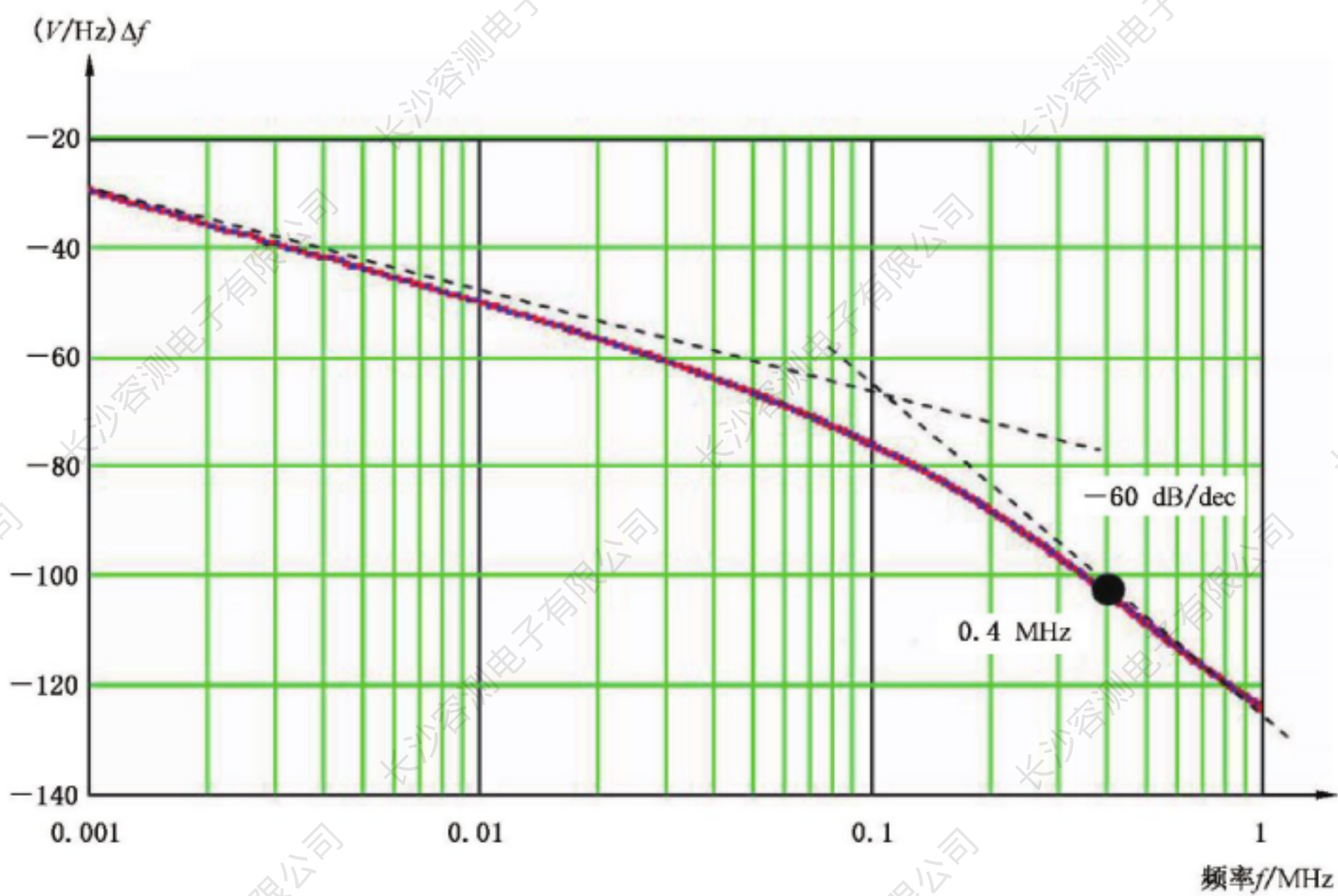
图 E.9 浪涌电压(10/700 \mu s):频域响应图, \Delta f = 0.2 kHz
