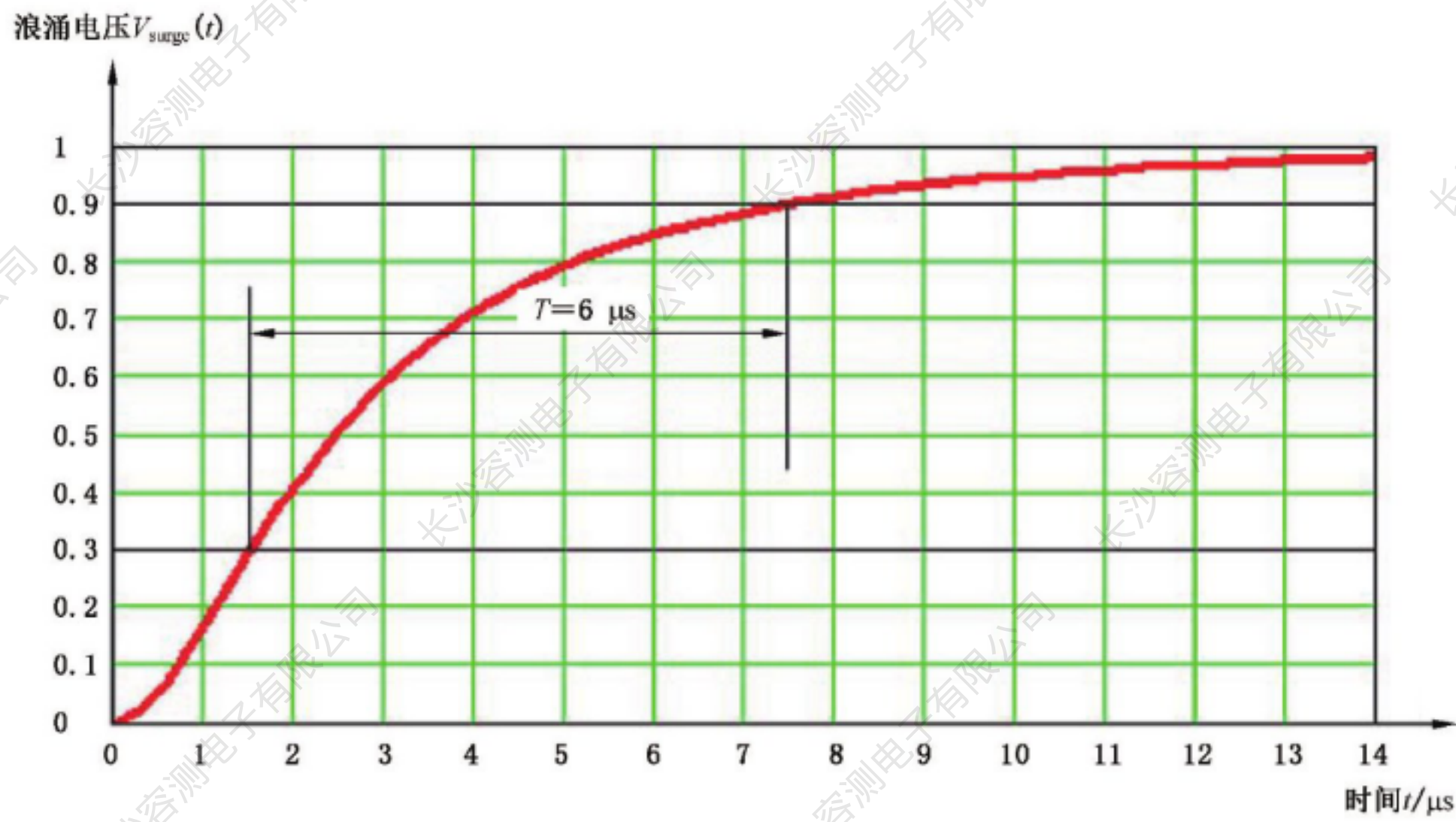
图 E.8 浪涌电压(10/700 \mu s):上升时间 T
